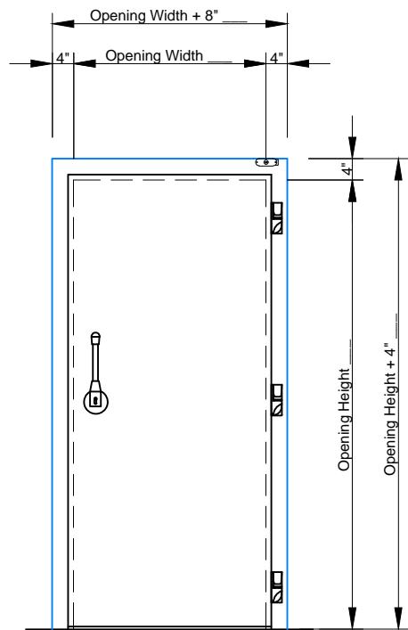
① SCALE: 3/8" = 1'-0"
